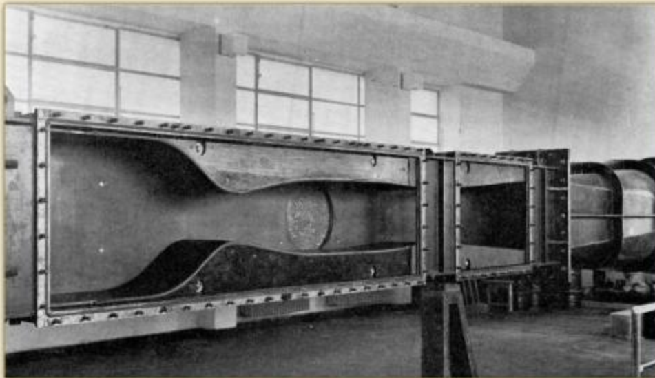
Sotto: Il condotto di trasformazione della galleria ultrasonica.
